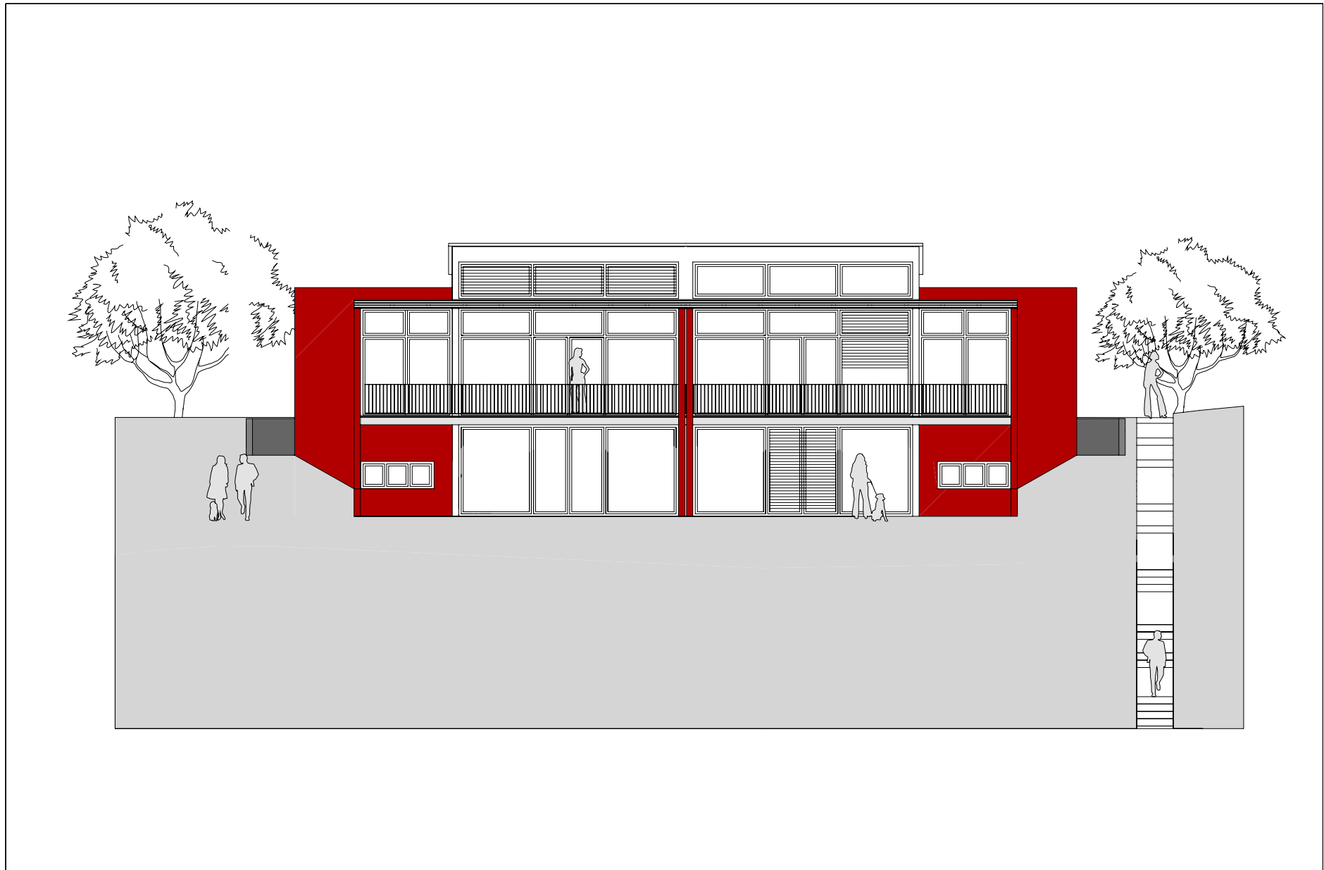
ANSICHT NORD-WEST
