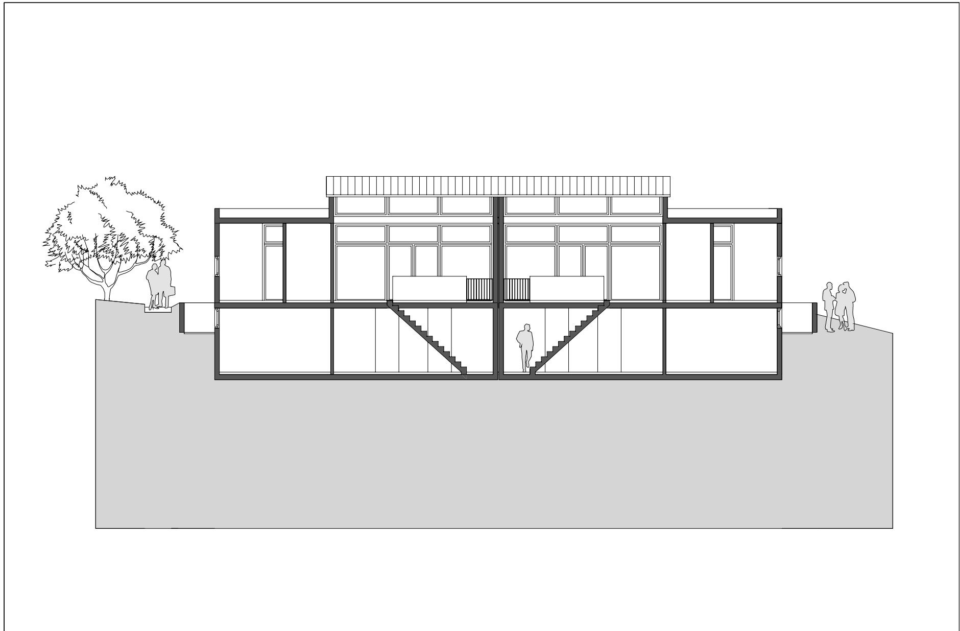
LÄNGSSCHNITT B-B
