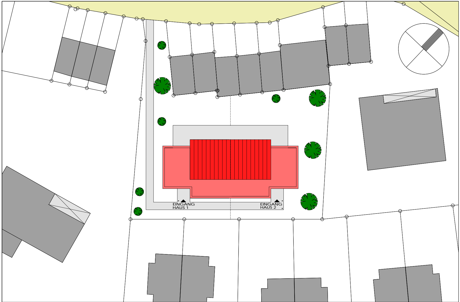
LAGEPLAN
